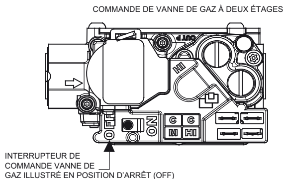
Fig. 11 – Interrupteur de commande en position d'arrêt (OFF)
