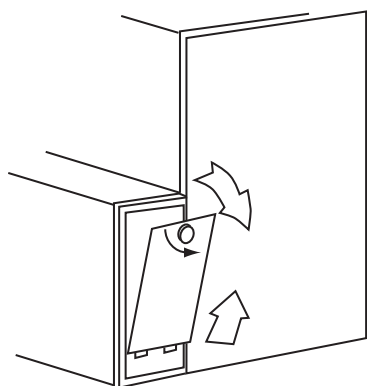
Fig. 21 – Retrait de la porte du boîtier de filtre de soufflante latérale
