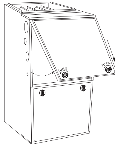
Fig. 10 – Retirez la porte principale de la chaudière (configuration à tirage ascendant)
