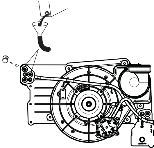
Fig. 30 – Protection de la chaudière contre le froid
