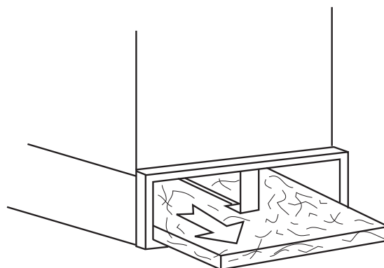
Fig. 24 – Retrait du filtre du boîtier de filtre de soufflante par le bas
