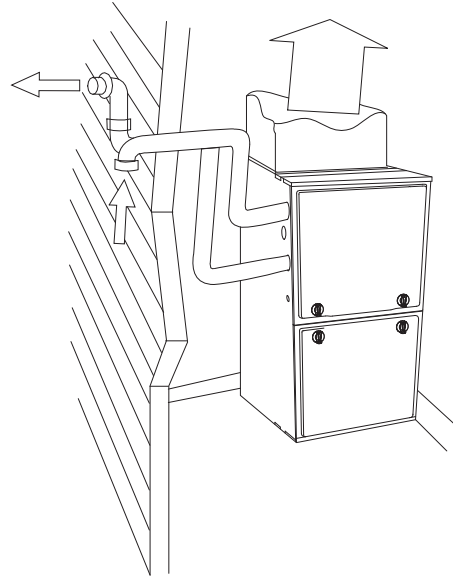
Fig. 2 – Tuyaux d'évent extérieurs
