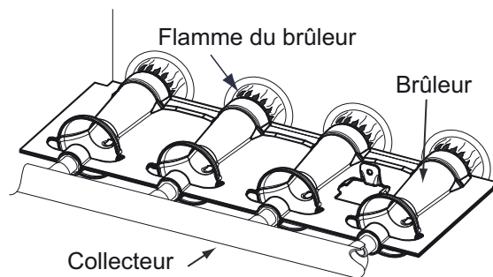
Fig. 5 – Réglage de la flamme des brûleurs
