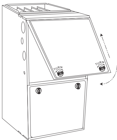
Fig. 13 – Panneau de service de la chaudière remis en place (configuration à tirage ascendant)
