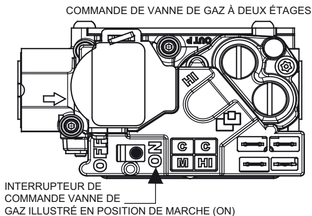
Fig. 12 – Interrupteur de commande en position de marche (ON)
