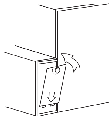
Fig. 25 – Remplacement de la porte du boîtier de filtre de soufflante latérale
