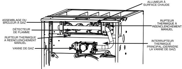
Fig. 27 – Ensemble de brûleurs à gaz (tirage ascendant)
