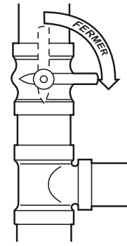
Fig. 8 – Fermez le robinet
