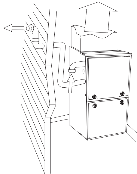
Fig. 3 – Tuyau d'air de combustion intérieur
