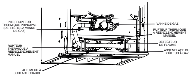
Fig. 28 – Ensemble de brûleurs à gaz (tirage descendant)
